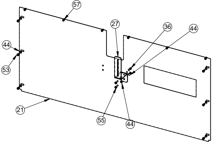
Eclaté A
