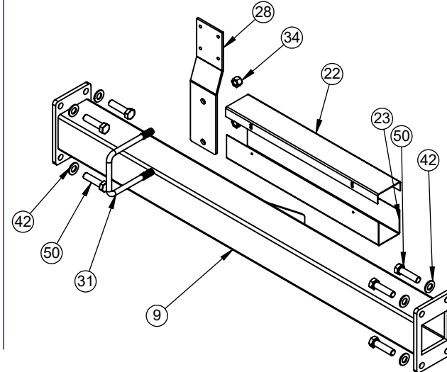
Eclaté F
