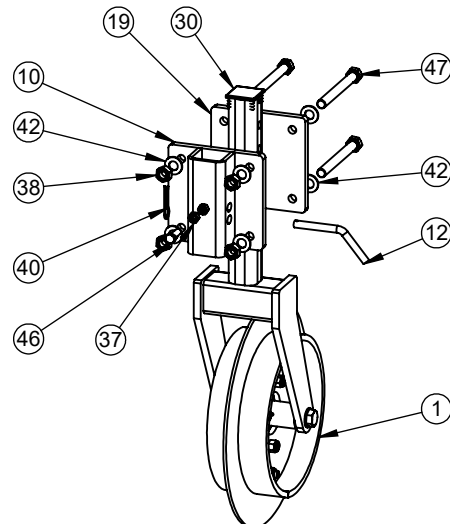
Eclaté E qte 2
