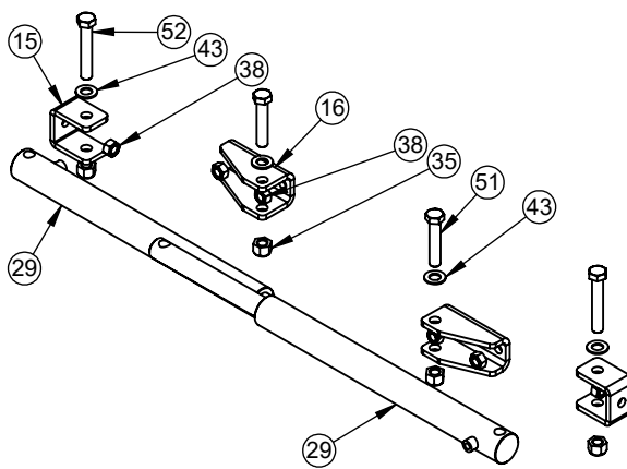
Eclaté D
