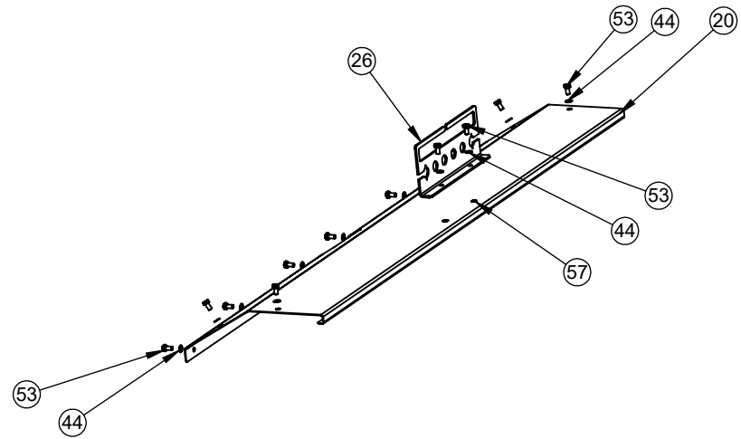
Eclaté H
