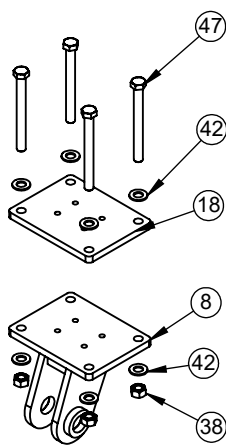
Eclaté B qte 2
