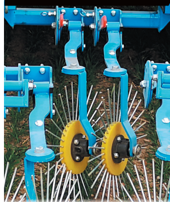
Rotors centraux de recouvrement (de série)
